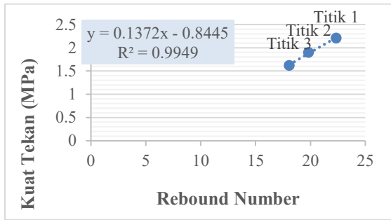
Gambar 2. Grafik Korelasi rebound number dengan kuat tekan (UCS)
