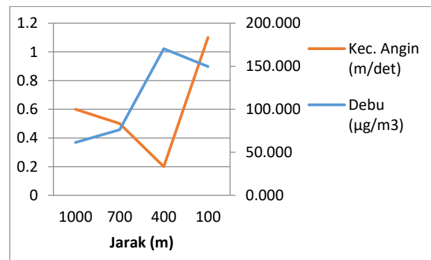
Gambar 1. Grafik Hubungan Kecepatan Angin vs Konsentrasi Debu di Pagi Hari
