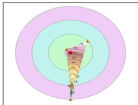
Gambar 8. Pola Dispersi Konsentrasi Debu di Pagi Hari
