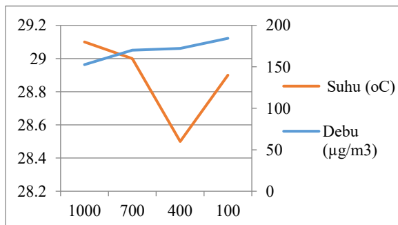
Gambar 5. Grafik Hubungan Suhu vs Konsentrasi Debu di Siang Hari
