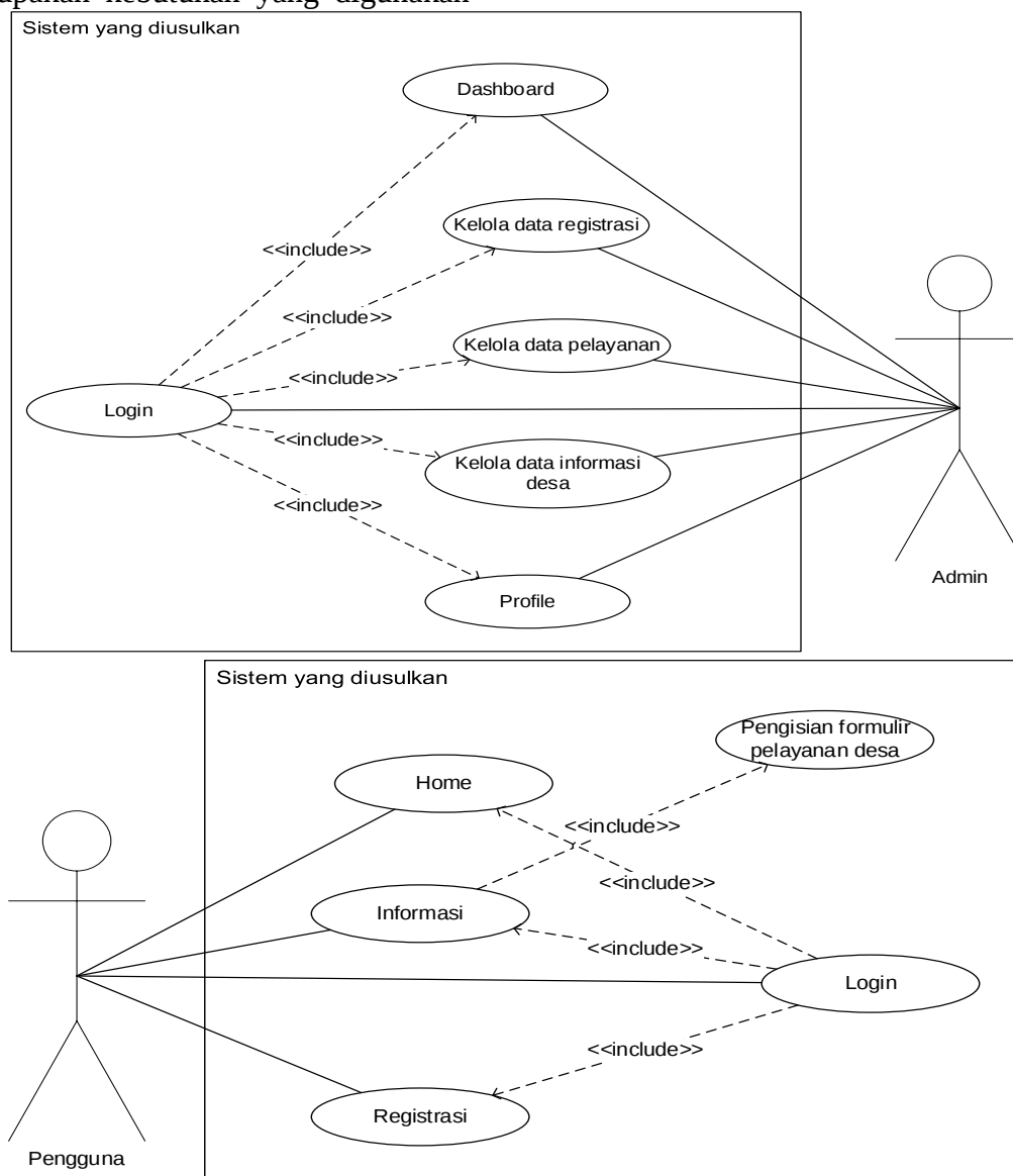
Gambar 1. Use Case Diagram Admin (atas) dan User (bawah)
