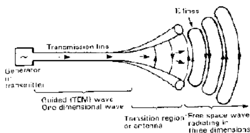
Gambar 1. Konsep dasar antena [1]
