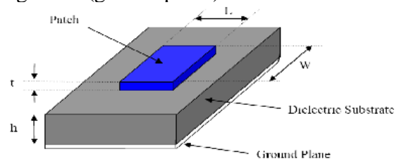
Gambar 2. Antena Mikrostrip
