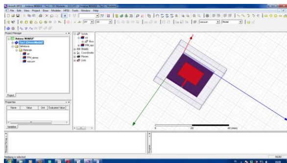
Gambar 1. Desain Antena Mikrostrip
